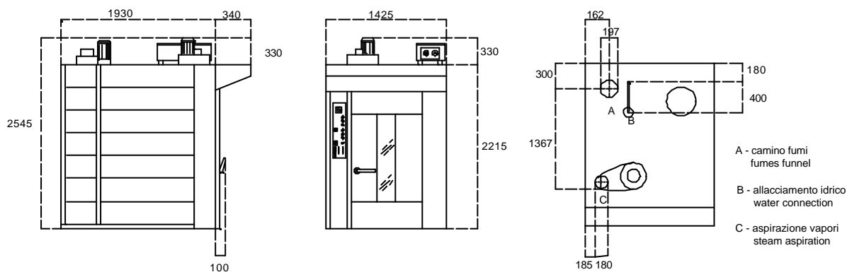
ROTOR mod. 68
