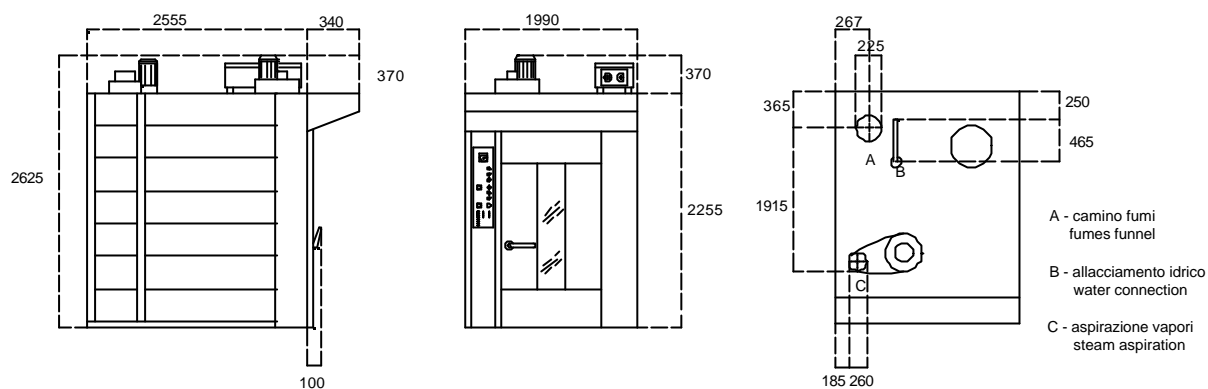
ROTOR mod. 812
